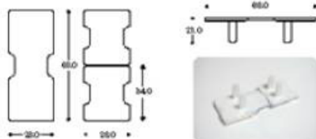
上面図
