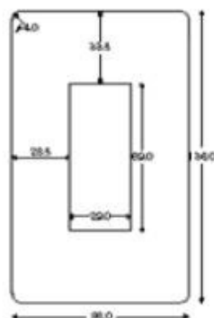
上面図 (平板)
